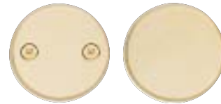
Peitekilpi 029 Materiaali: messinki. Pintakäsittely: kiillotettu Ms/KILA, kromattu Ms/CR, harjattu Ms/HA, oksidoitu Ms/OKS, valkoinen Ms/JVA, satiinikromattu Ms/HCR.
